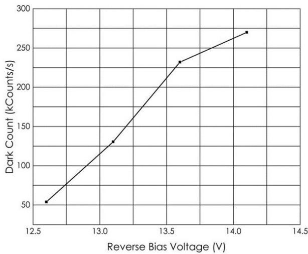
暗计数 vs. 反向偏置电压
