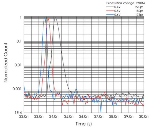
时间抖动
